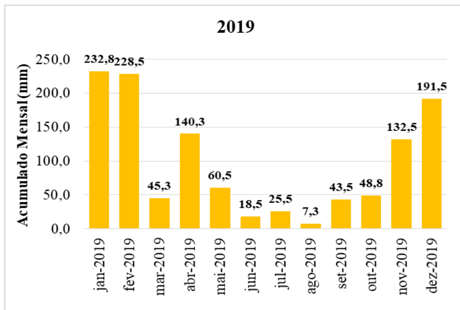
Precipitação mensal acumulada (mm) do pluviógrafo P2 no ano de 2019 (dados atualizados até 31/12/19).
