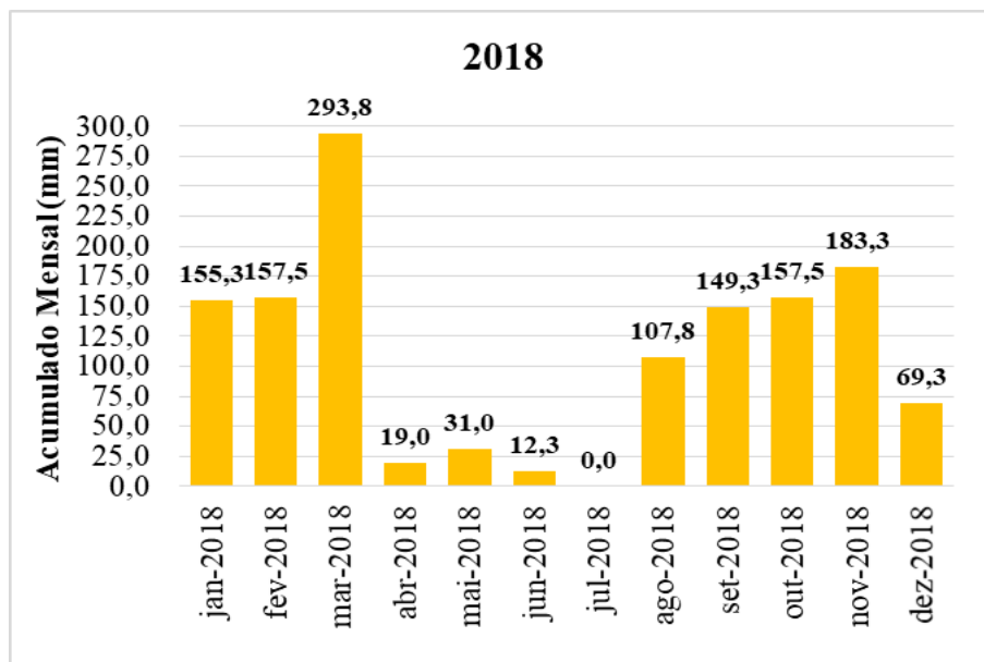
Precipitação mensal acumulada (mm) do pluviógrafo P2 no ano de 2018.
